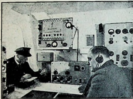
Fig. 2. De nieuwe kortegolfinstallatie van de „Graf Zeppelin”. Midden boven: de 50 watt kortegolfzender van Telefunken. Midden onder: de ontvanger. Rechts: de peilontvanger.
